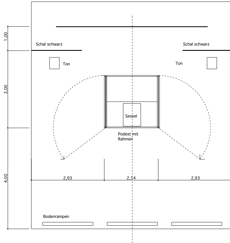
Grundriss Der tollste Tag M. 1:50
